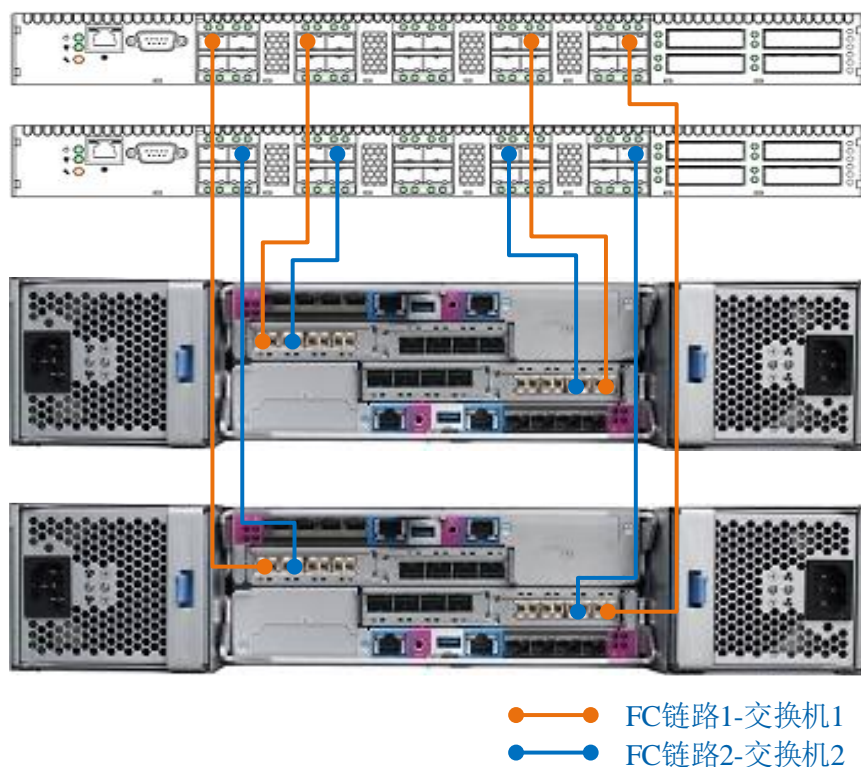
图 2-1 四个控制器冗余连接方式（2U NVMe 控制柜）
