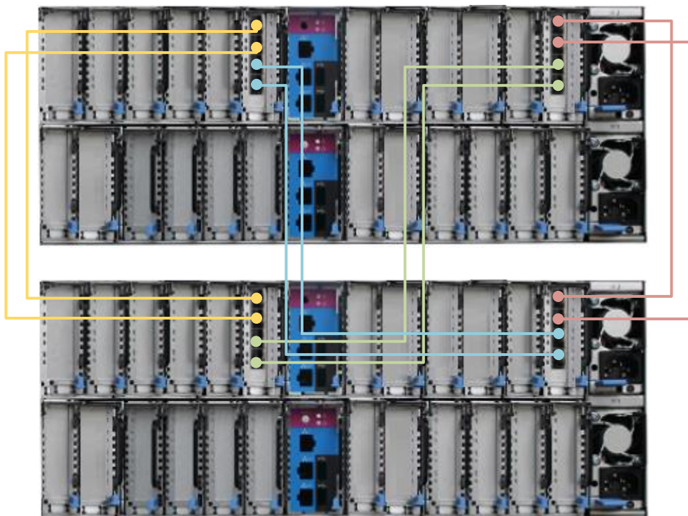
图 2-5 通过 NTB 卡四控连接-单端口线缆方式 1
