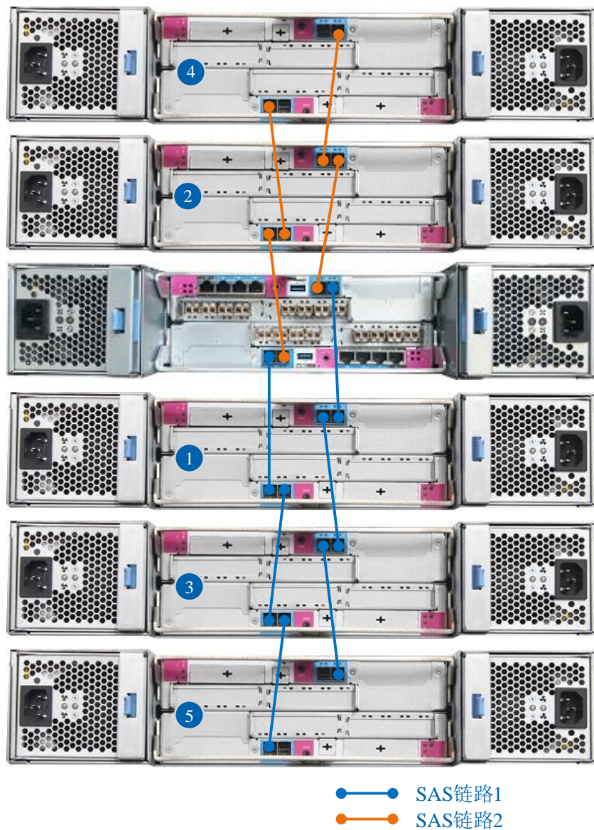
图 2-9 连接 5 台扩展柜 (2U SAS 控制柜不使用 SAS 卡)
