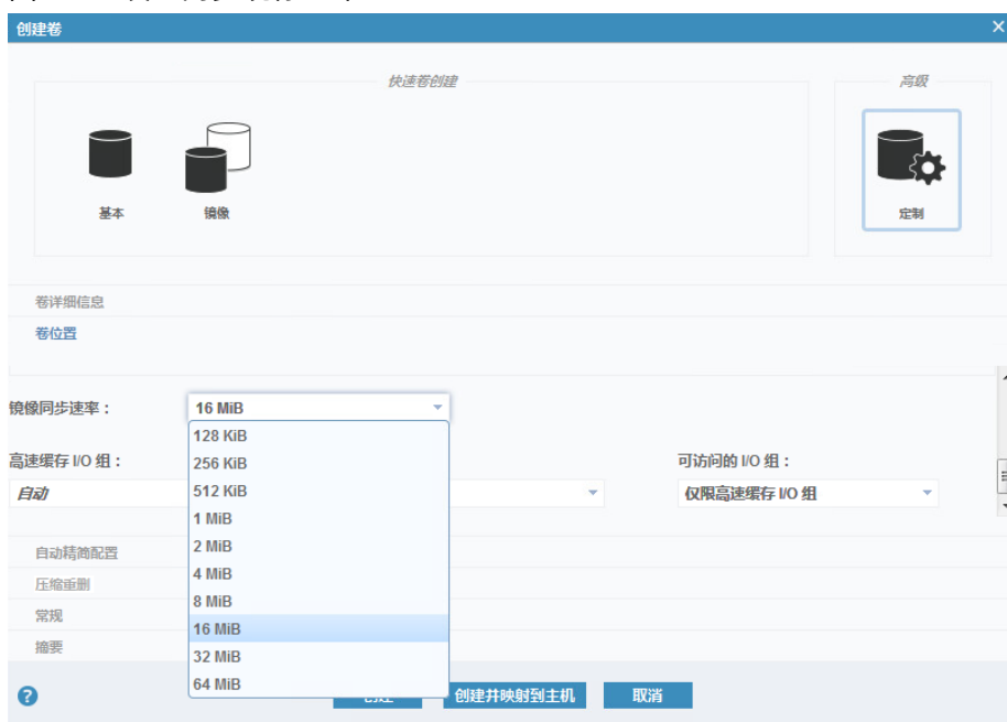
图 6-20 设置同步镜像速率
