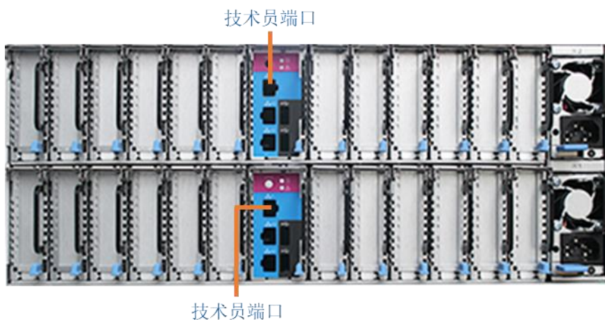
图 3-10 技术员端口（4U 控制柜）
