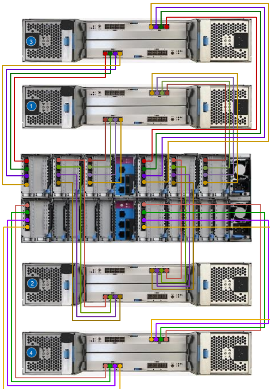
图 2-14 无 ACC 时连接 JBOF 扩展柜（4U 控制柜）
