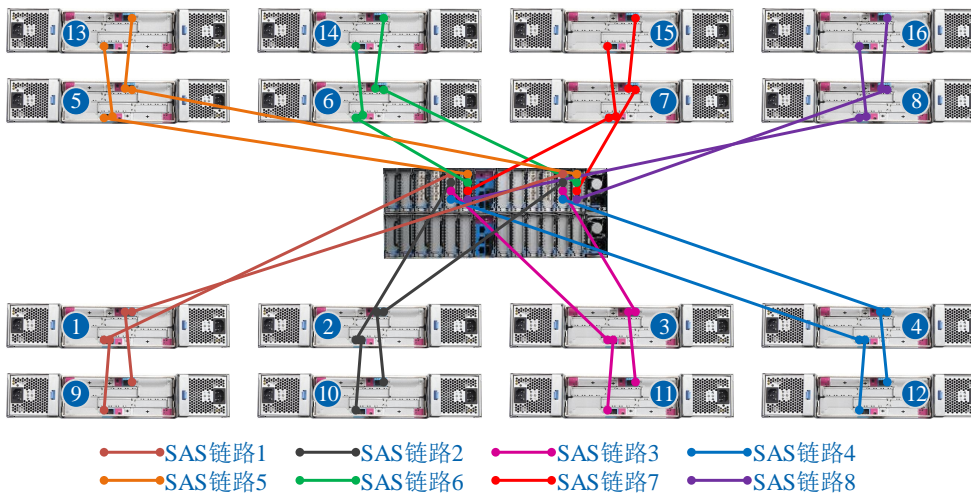
图 2-11 连接 16 台扩展柜（4U 控制柜使用 2 个 4 口 SAS 卡）
