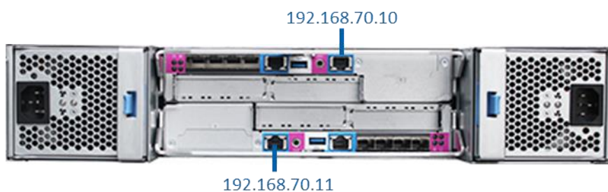
图 3-1 已设置服务 IP 的端口 1 位置（2U NVMe 控制柜）
