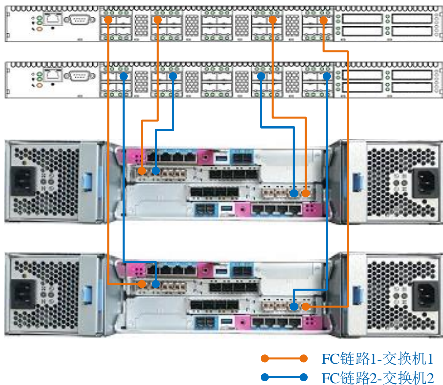
图 2-2 四个控制器冗余连接方式（2U SAS 控制柜）
