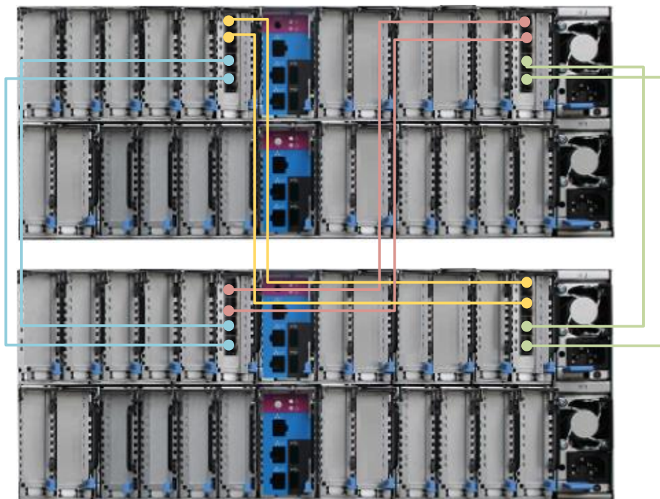
图 2-6 通过 NTB 卡四控连接-单端口线缆方式 2
