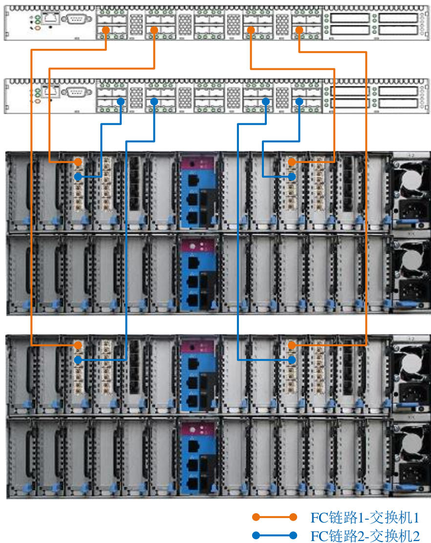
图 2-7 四个控制器冗余连接方式（4U 控制柜）
