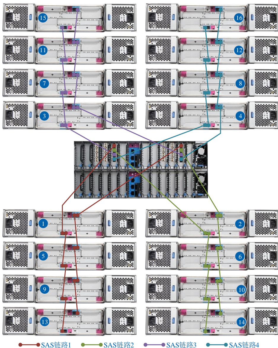
图 2-12 连接 16 台扩展柜（4U 控制柜使用 1 个 4 口 SAS 卡）
