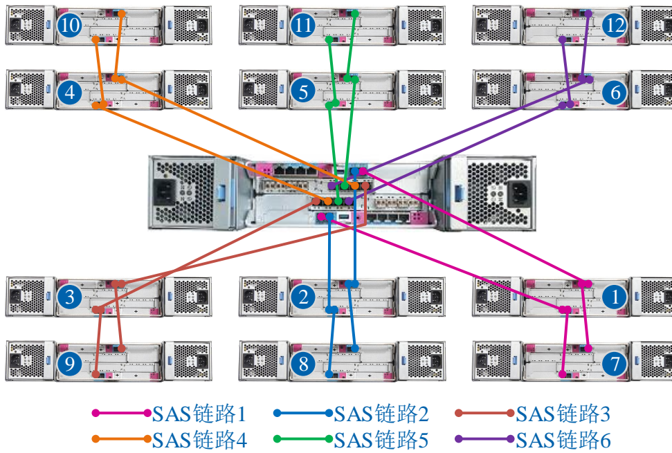
图 2-10 连接 12 台扩展柜（2U SAS 控制柜使用 SAS 卡）
