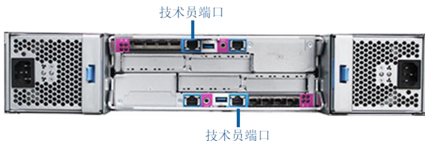
图 3-8 技术员端口（2U NVMe 控制柜）
