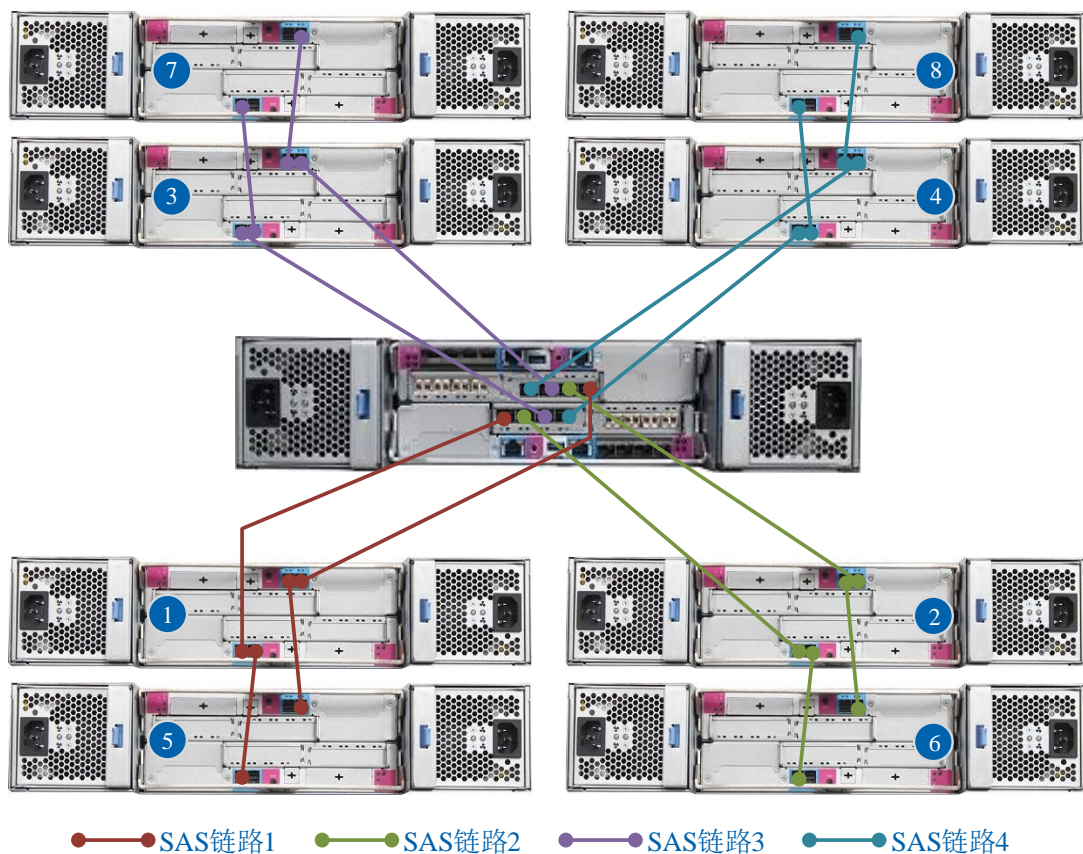
图 2-8 连接 8 个扩展柜（2U NVMe 控制柜）
