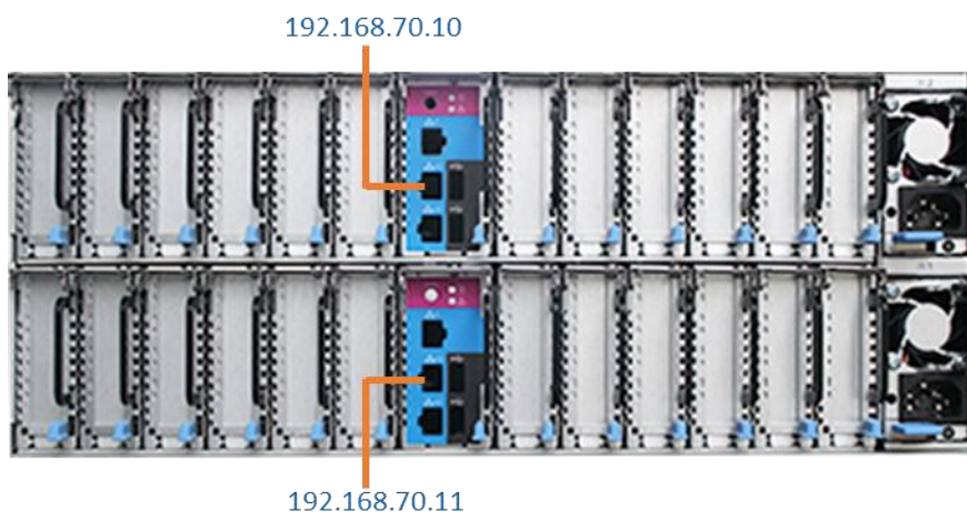
图 3-3 已设置服务 IP 的端口 1 位置（4U 控制柜）
